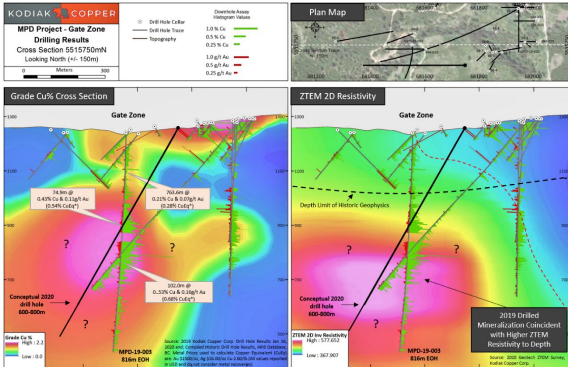
Abbildung 1 - Gate Zone: Querschnitte der historischen Bohrungen, Kodiaks Bohrloch MPD 19-003 und die anhand der ZTEM-2D-Messung neu entdeckte Zone mit hohen Widerständen. Das linke Bild zeigt eine Farbkonturierung zur Darstellung des Kupfergehalts; die Farbbalken repräsentieren den Kupfergehalt in Prozent (grün) und den Goldgehalt in Gramm/Tonne (rot) im Kern. Das rechte Bild ist eine Farbkonturierung im 2D-Format; es zeigt einen Querschnitt der Zone mit hohen Widerständen, die anhand der aktuellen luftgestützten ZTEM-Messung ermittelt wurde.
