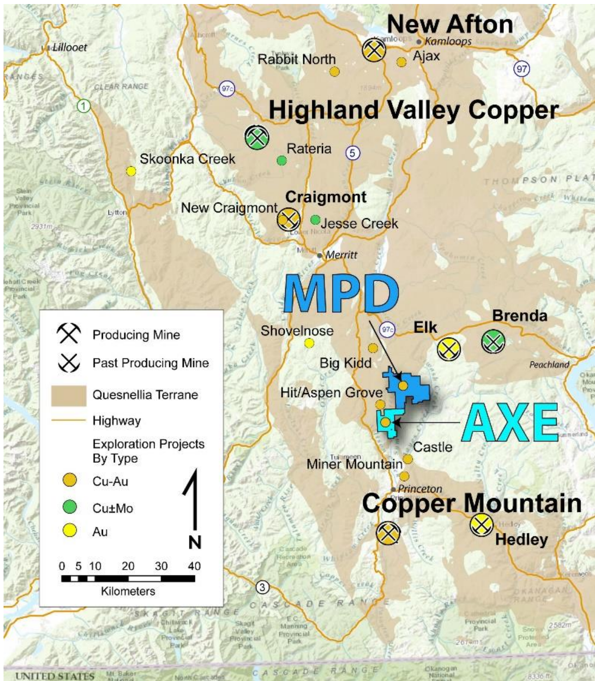
Abbildung 1: Lageplan, MPD-Axe-Liegenschaften
