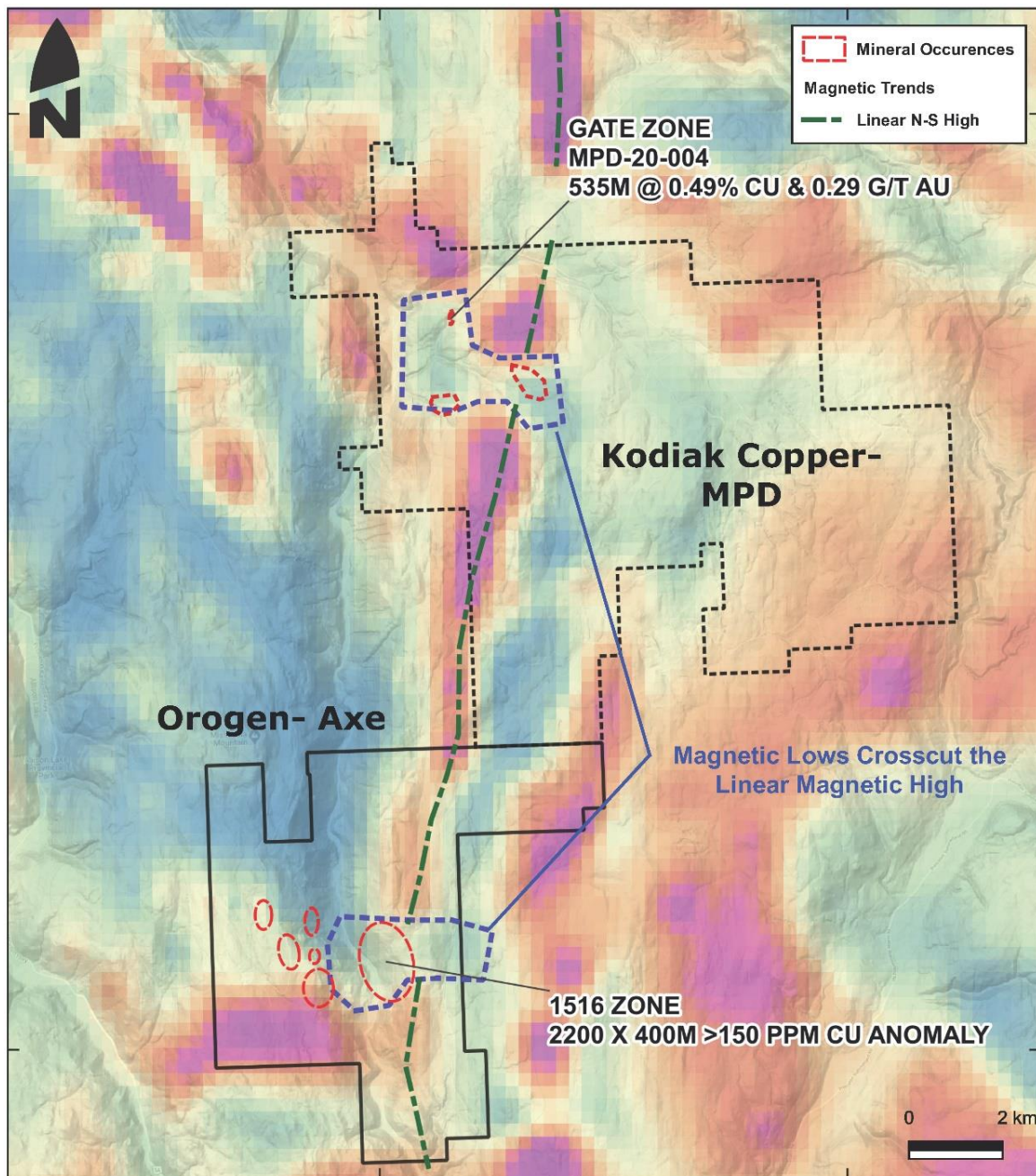
Abbildung 3: Lage der Zonen 1516 und Gate, magnetische Gesamtintensität
