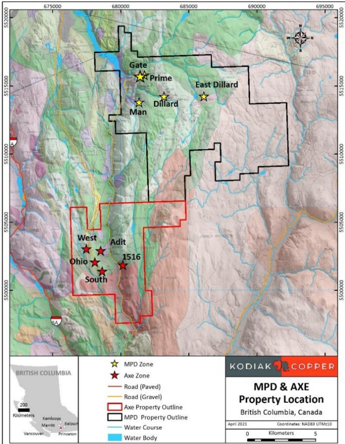
Abbildung 2: Geologie und Kupfer-Porphyr-Zonen, MPD-Axe-Liegenschaften
